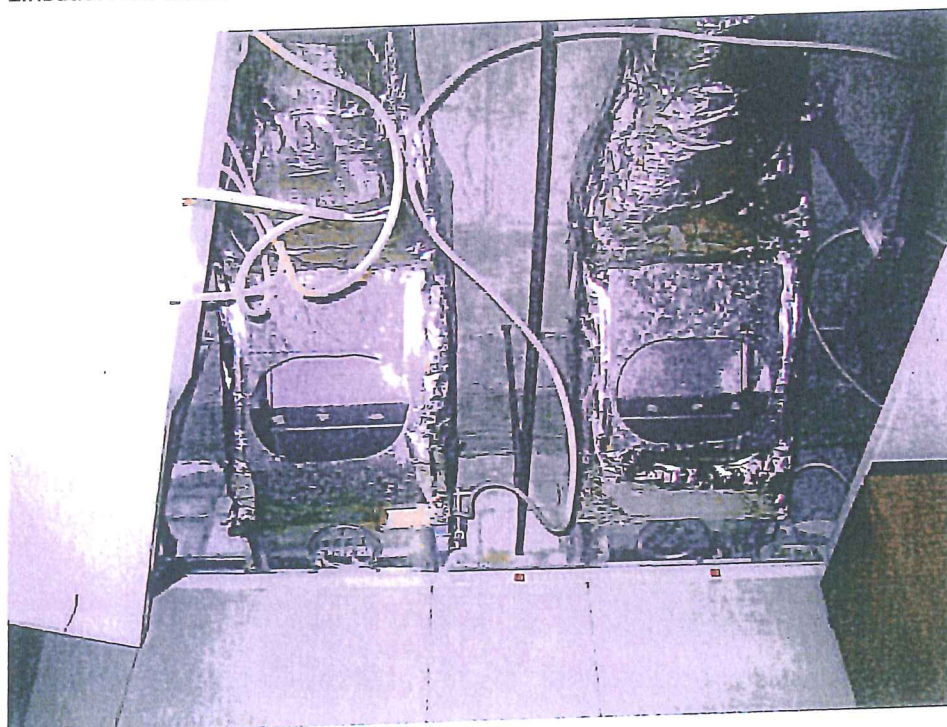
Einbauort der sanierten Brandschutzklappen (Bürräume)
